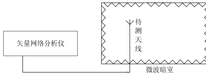
图2 天线信号频率范围、输入电压驻波比测试框图
